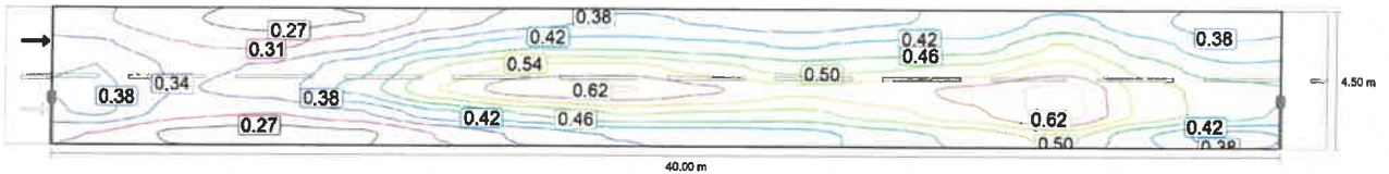
Observator 2: Densitatea luminii la instalația nouă [cd/m 2 ] (Linii Isolux)
