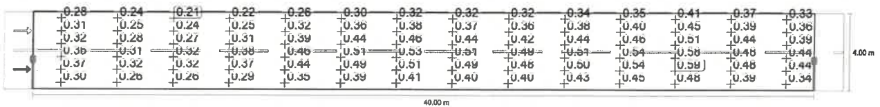
Observator 1: Valoarea de întreținere, densitatea luminii cu carosabil uscat [cd/m 2 ] (Raster valoric)
