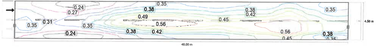
Observator 2: Valoarea de întreținere, densitatea luminii cu carosabil uscat [cd/m 2 ] (Linii Isolux)
