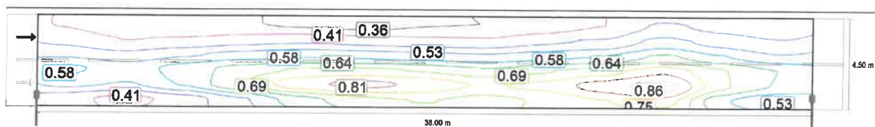
Observator 2: Valoarea de întreținere, densitatea luminii cu carosabil uscat [cd/m²] (Linii Isolux)
